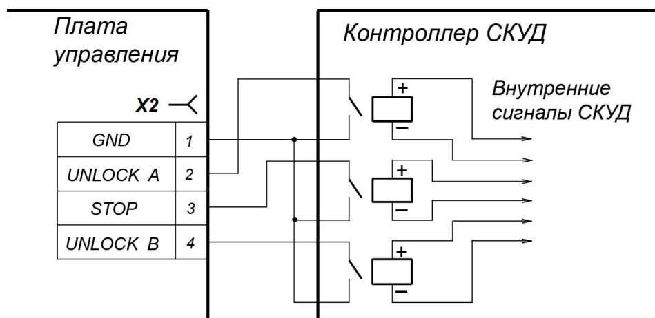
Рисунок 12. Управляющие элементы внешнего устройства – нормально разомкнутый контакт реле
