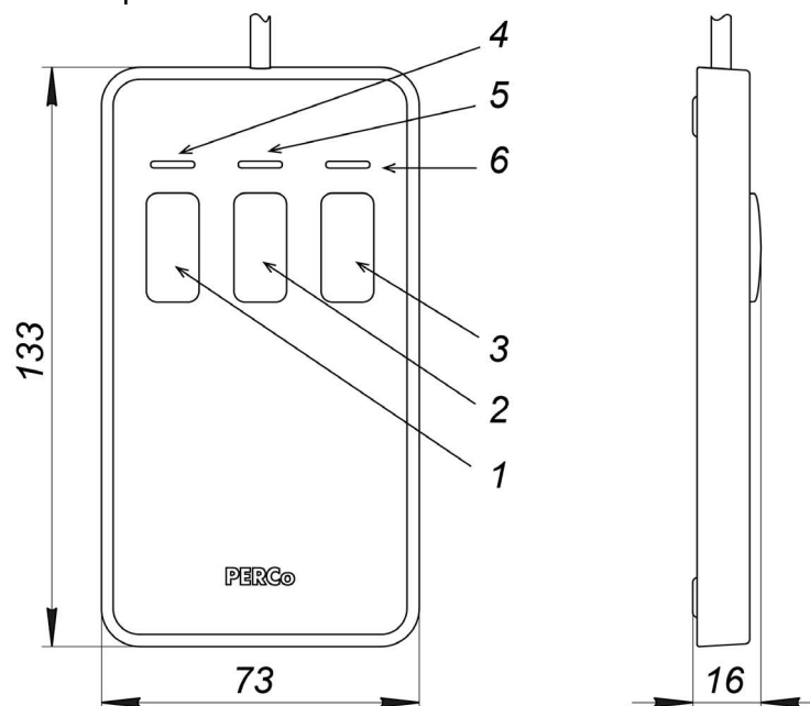
Рисунок 10. Общий вид и габаритные размеры ПДУ:
