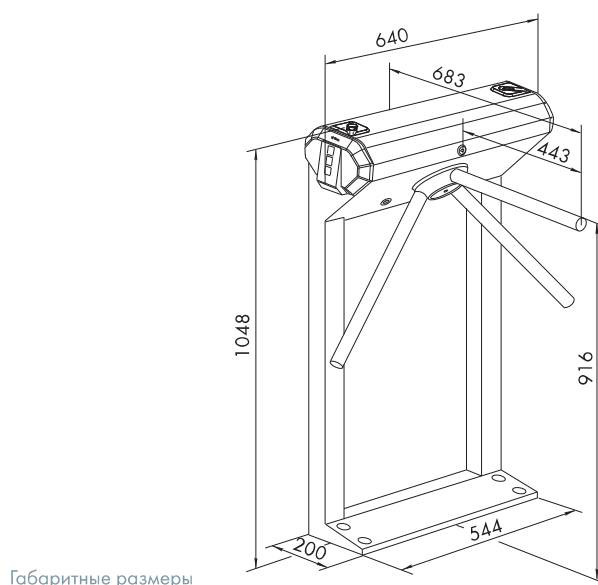
Габаритные размеры
