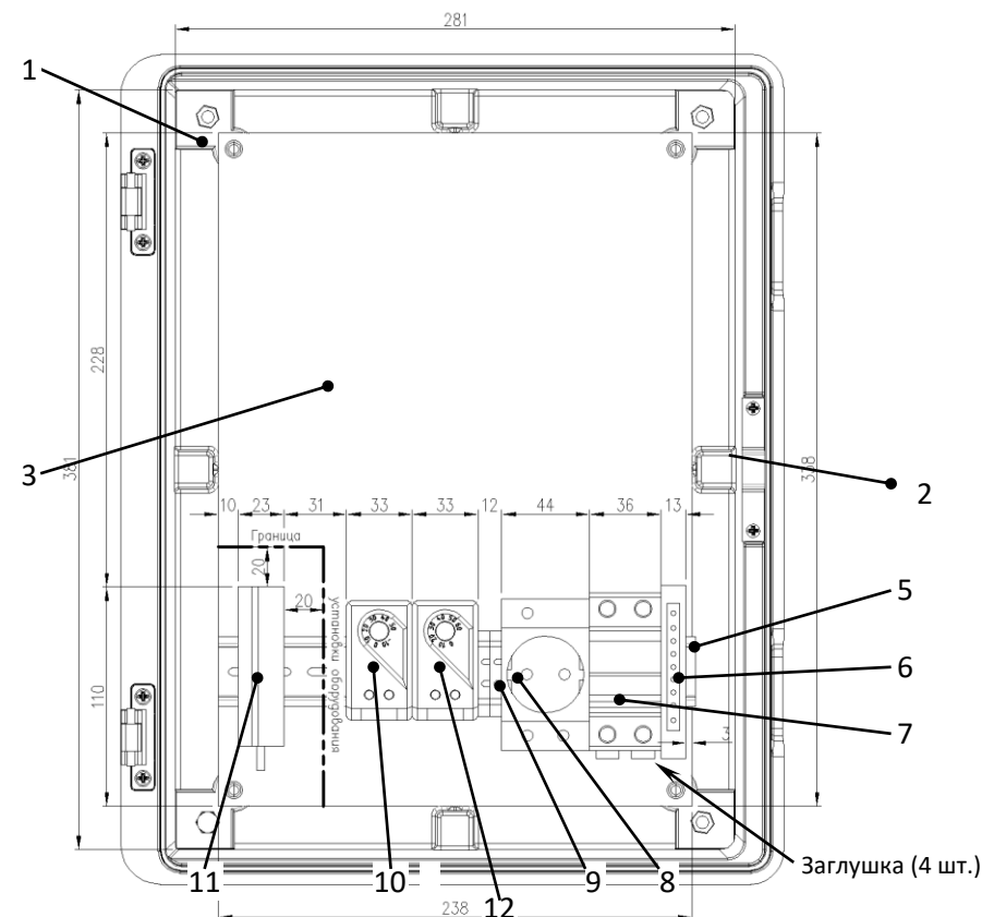
Рисунок 1 – Устройство шкафа
