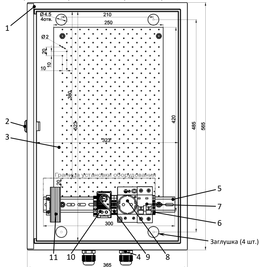
Рисунок 1 – Устройство шкафа
