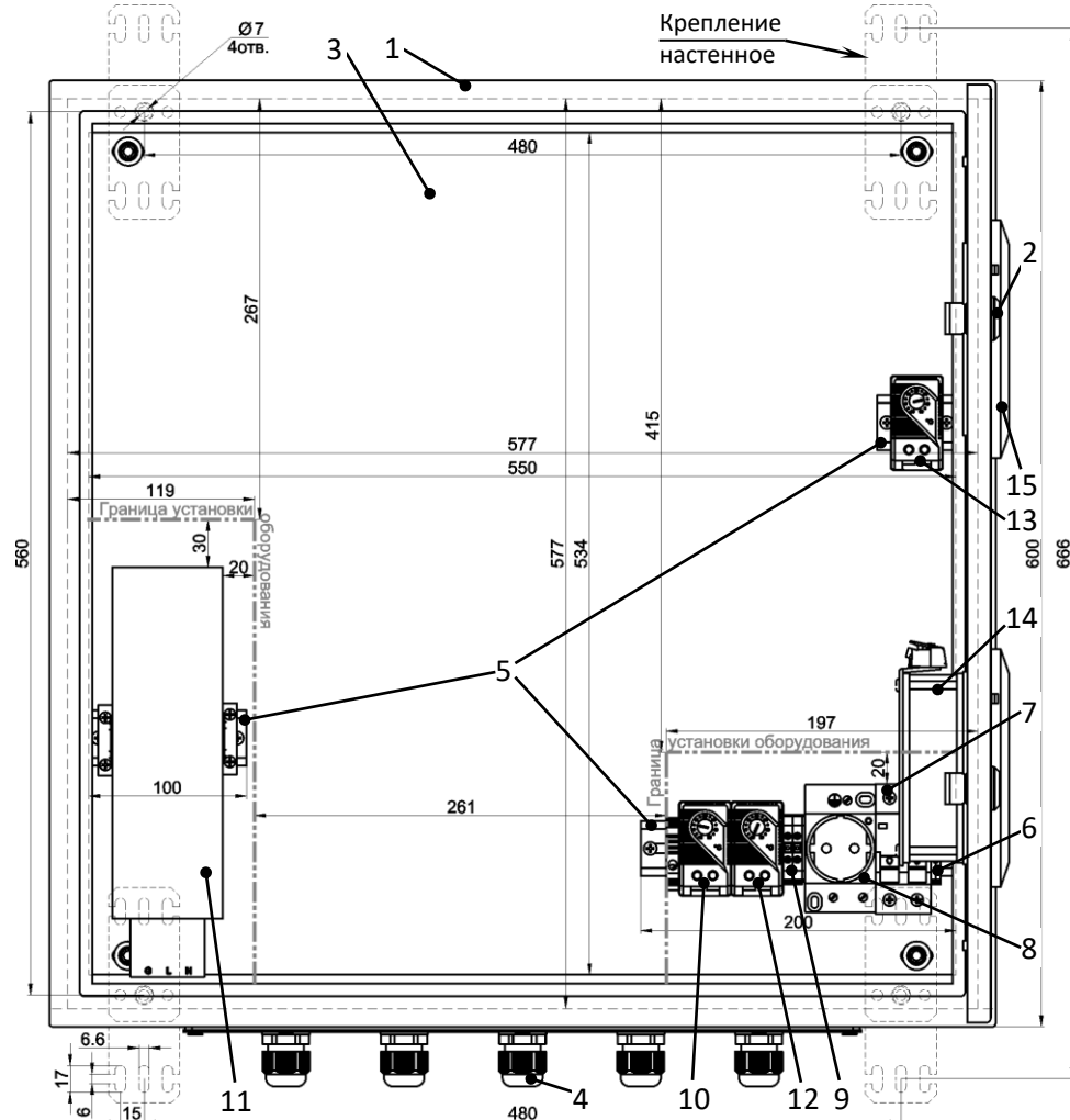
Рисунок 1 – Устройство шкафа
